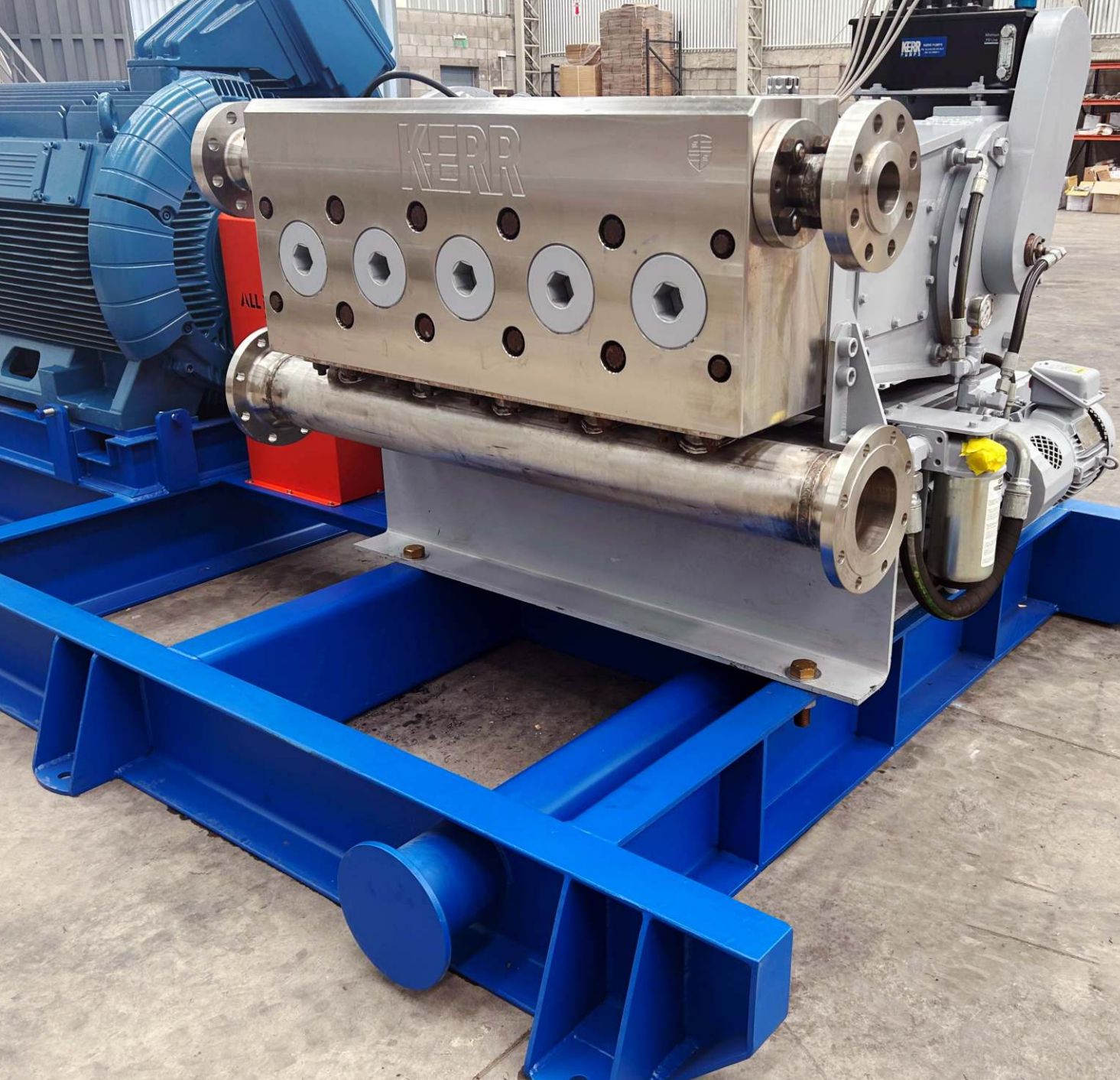
Opciones de bombas de triple y quintuple pistón para bombeo de fluidos a altas presiones.
